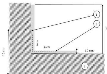
Figure 1. Relevé armé sur acrotère haut
