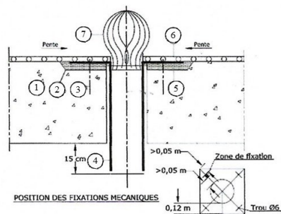
Figure 1 - Exemple de traitement d'une évacuation d'eau pluviale avec platine
